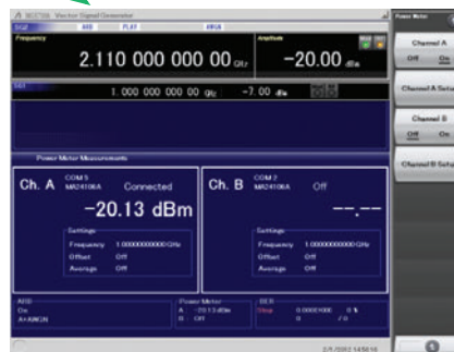
Power Meter Function
